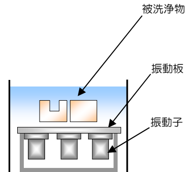
《振動板方式》
